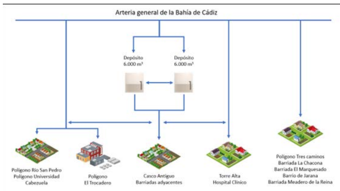
Figura 25. Esquema general de la zona de abastecimiento de Puerto Real. Fuente: Elaboración propia a partir del Protocolo de autocontrol y gestión de las redes de abastecimiento de Puerto Real.
