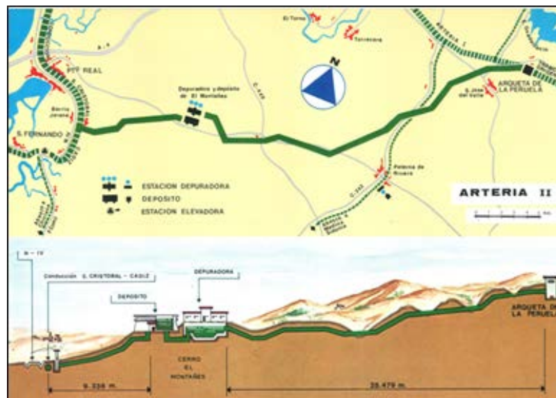
Figura 23. Ubicación y esquema del tramo II (Ramal Norte). Fuente: página web del CAZG.
